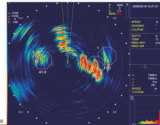
魚群追尾と魚量推定値機能
